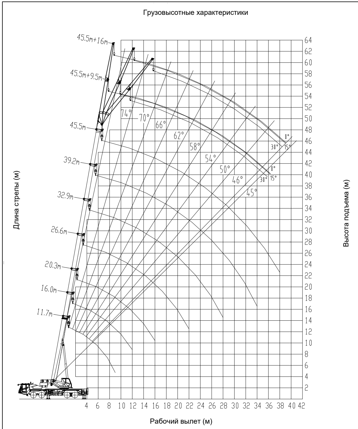
Рисунок 1 Грузовысотные характеристики
